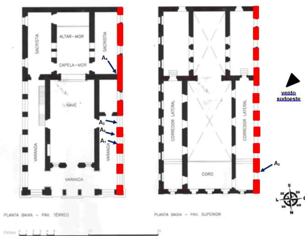
Figura 12: Plantas baixas do pavimento térreo e superior da Igreja da Comandaroba com a determinação do local e recolha das amostras A 1 , A 2 , A 3 , A 4 e A 5 na fachada oeste (em vermelho nas plantas baixas). Fonte: Inventário Nacional de Bens Móveis Integrados – IPHAN, 2001, p. 03-04 – alterações Grupo de pesquisa PIBITI, mar. 2023.
