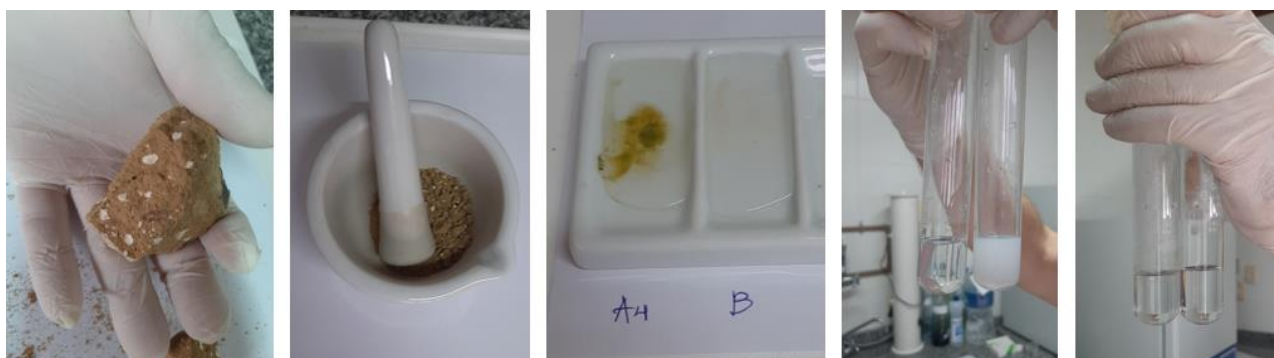
Figura 17: (da esquerda para direita) – Amostra A 4 após ser fracionada em dois pedaços mostrando as características de uma argamassa antiga (rica em nódulos de cal e em argila vermelha). Amostra A 4 sendo destorroada. Resultado ataque por Nitrato na amostra A 4 (alta concentração). Resultado do ataque por Cloreto na amostra A 4 (alta concentração). Resultado do ataque por Sulfato na amostra A 4 (inexistência). Fonte: Grupo de pesquisa PIBITI, jul. 2023.
