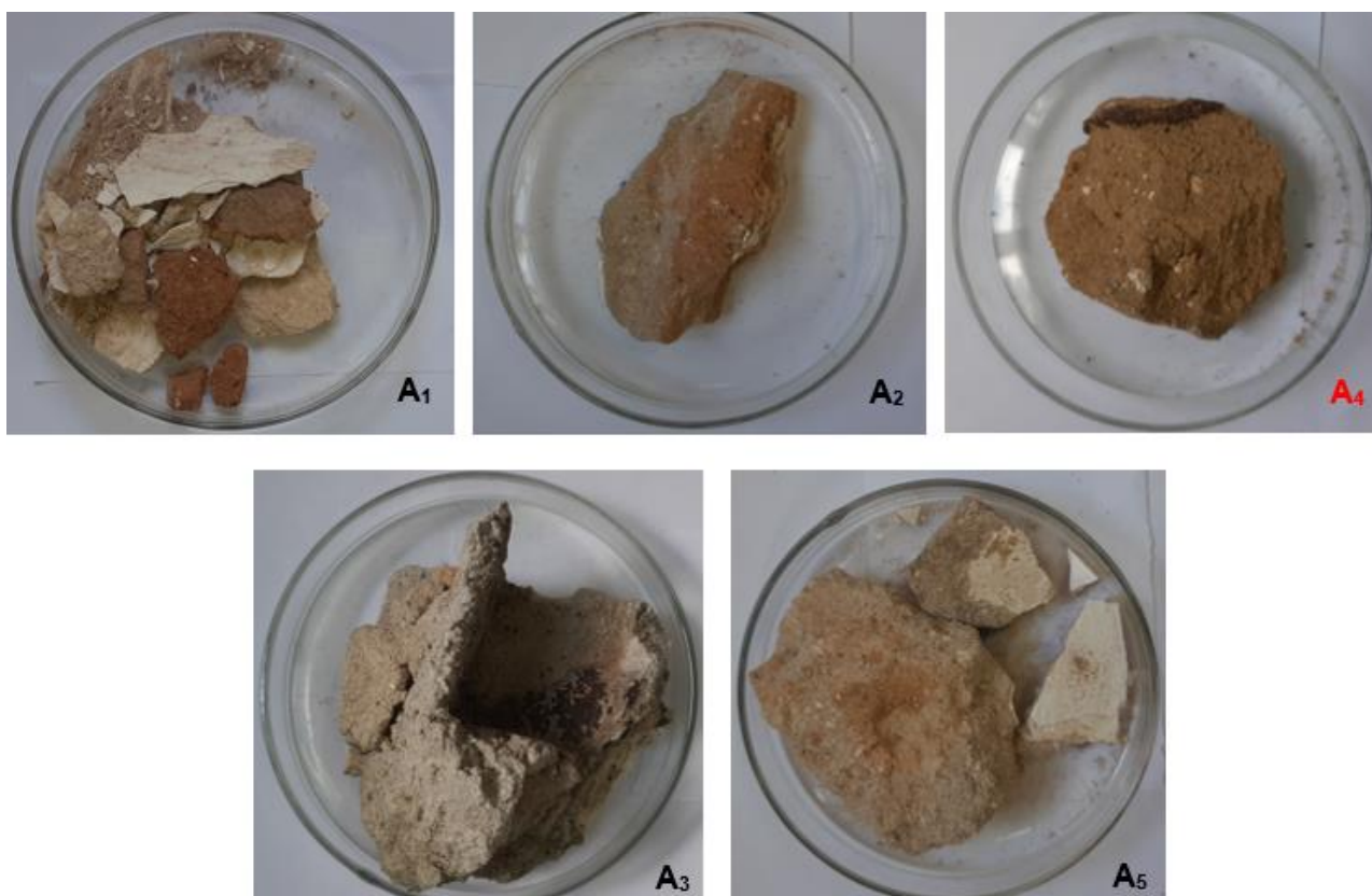
Figura 15: (acima – da esquerda para direita) – Amostras A 1 , A 2 e A 4 , esta última apesar de semelhanças com as anteriores é a que possui mais possibilidades de representar a argamassa “antiga” da Igreja da Comandaroba. (abaixo – da esquerda para a direita) – Amostras A 3 e A 5 presença de cimento – argamassa de complementação moderna. Fonte: Grupo de pesquisa PIBITI, jun. 2023.
