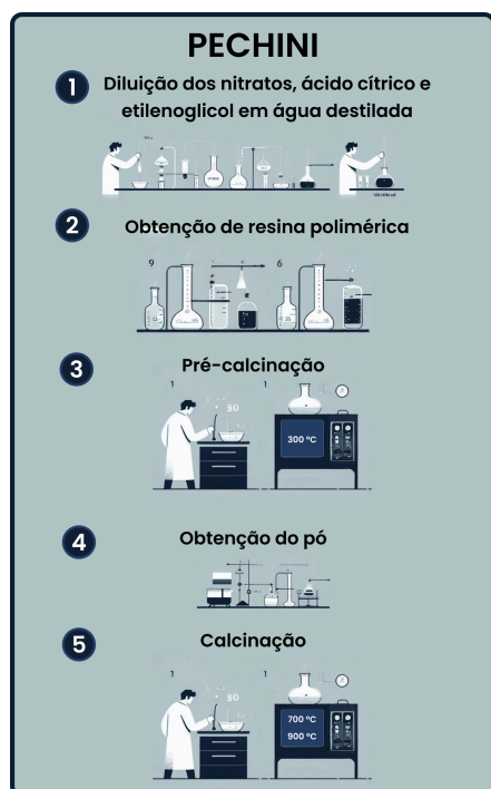
Figura 1. Fluxograma explicativo sobre o método Pechini
