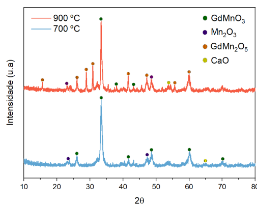
Figura 5. Difratogramas do catalisador de composição GD
