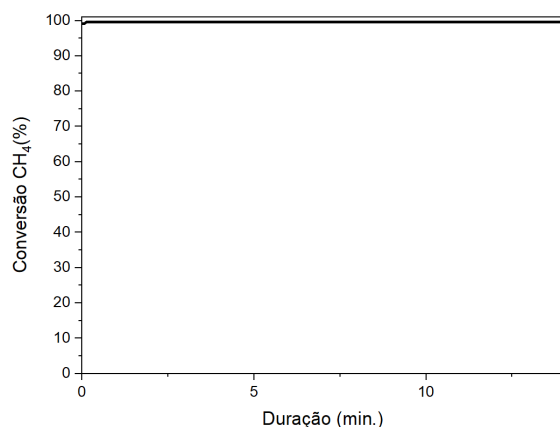
Figura 11. Curva de estabilidade do catalisador LA
