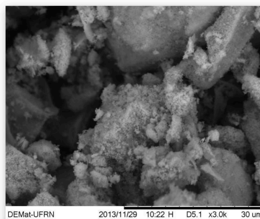
Figura 9. Micrografias do catalisador de composição GD na temperatura de 900 °C
