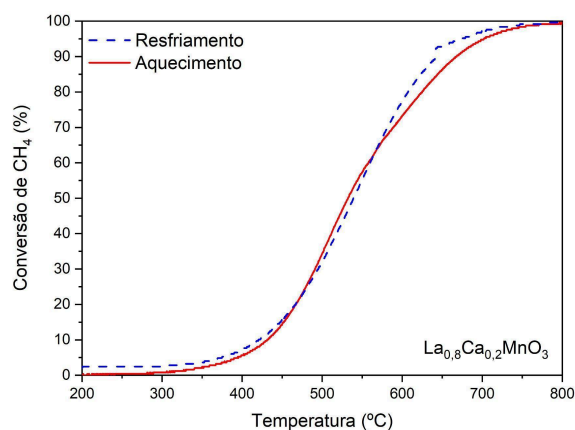
Figura 10. Curvas de resfriamento e aquecimento do catalisador LA
