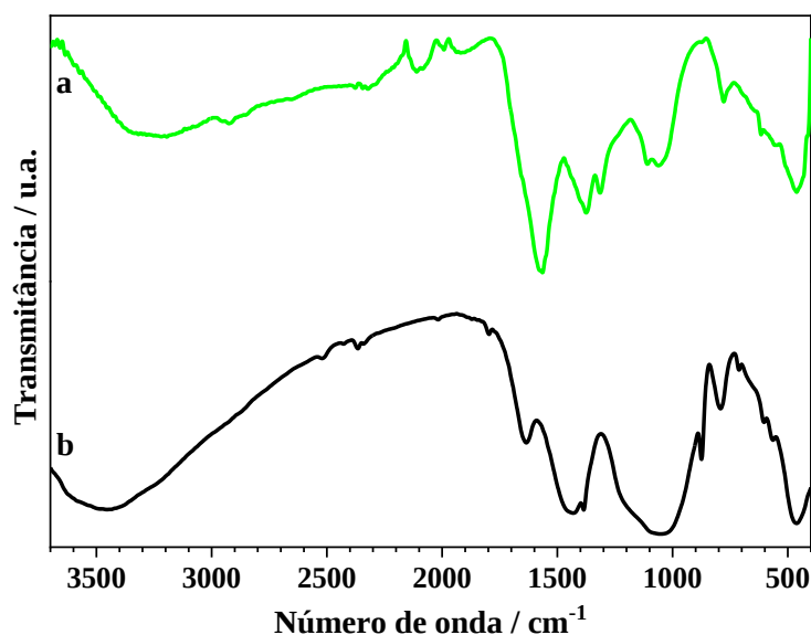
Figura 1. Espectro FTIR: (a) Cinzas da planta Equisetum hyemale , e (b) Compósito BGCarb.
