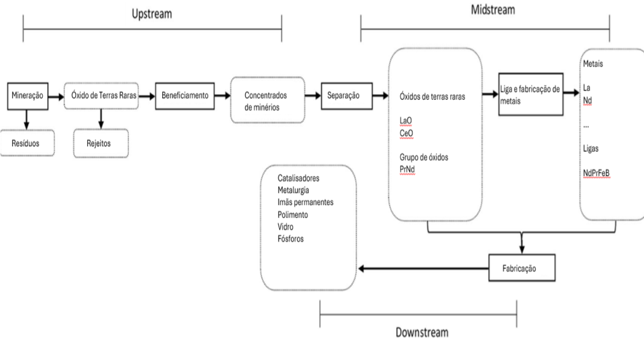
Figura 2 - Fluxograma da Cadeia Produtiva de Terras Raras
