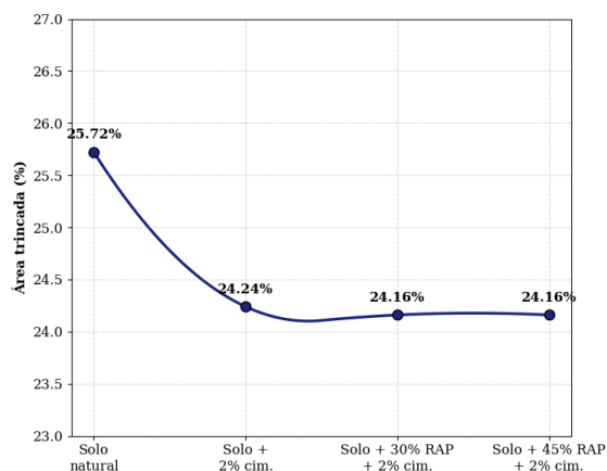
Figura 7. Tendência de área trincada das misturas.
