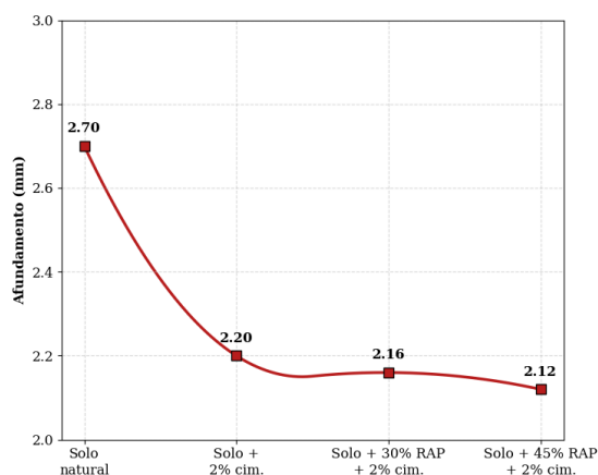
Figura 8. Tendência de afundamento das misturas.
