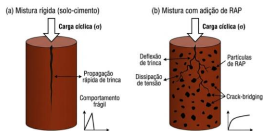
Figura 9. Representação esquemática do comportamento sob carga cíclica.
