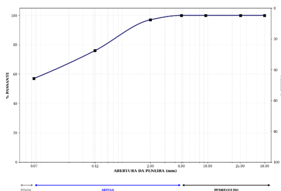
Figura 1. Curva granulométrica do solo natural.
