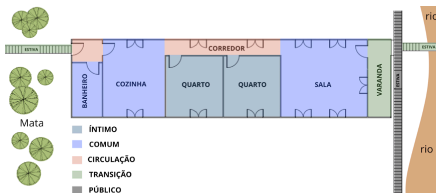
Planta baixa de tipologia mais comum dentre as casas do tipo palafita na comunidade estudada e de compreensão de situação espacial. Fonte: os autores, 2024
