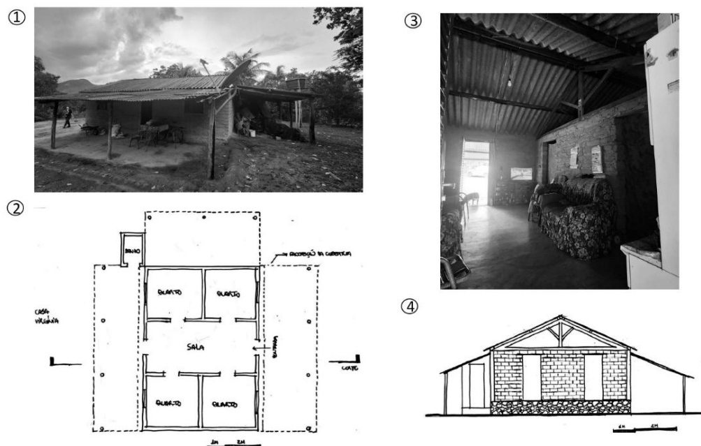
Figura 07: Imagem 1, imagem externa da casa; imagem 2 planta da casa de adobe; imagem 3, fotografia da parte interna da casa e imagem 4, corte da casa.
