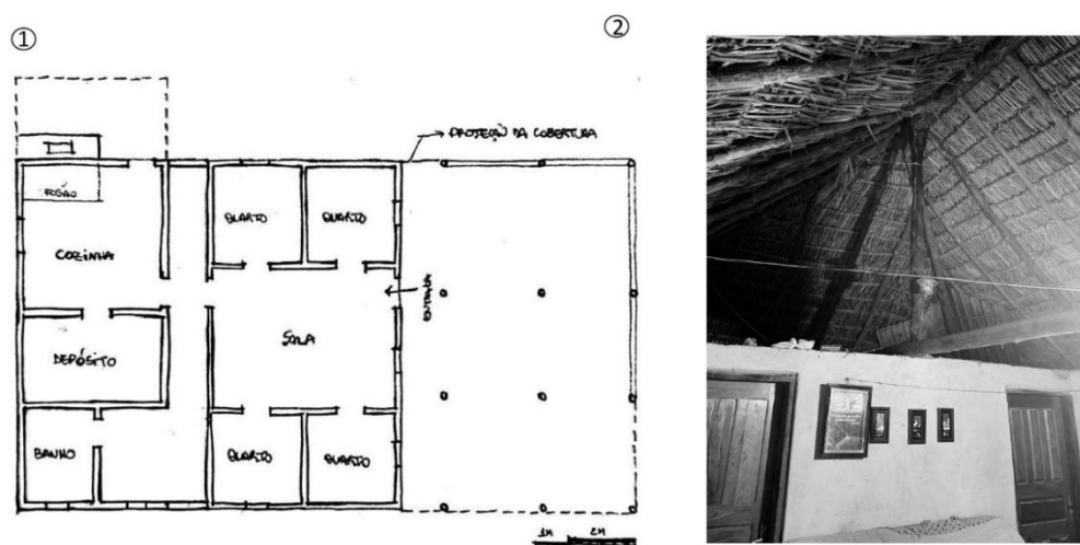
Figura 05: À esquerda, planta atual da casa de Dona Alvina e imagem interna da cobertura de fibra natural à direita.
